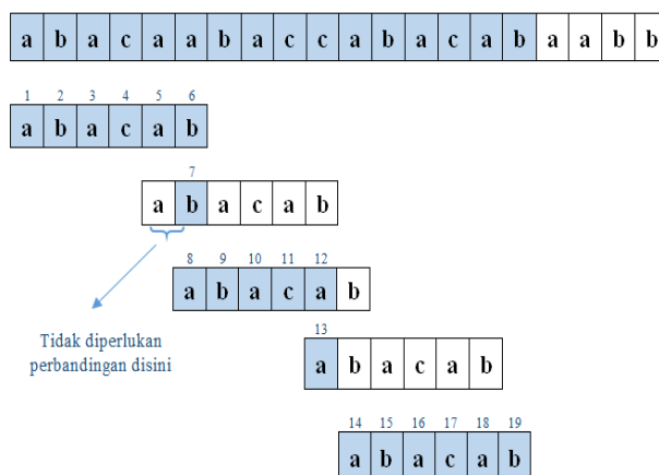
Gambar 1. Contoh eksekusi algoritma pencocokan pola KMP
